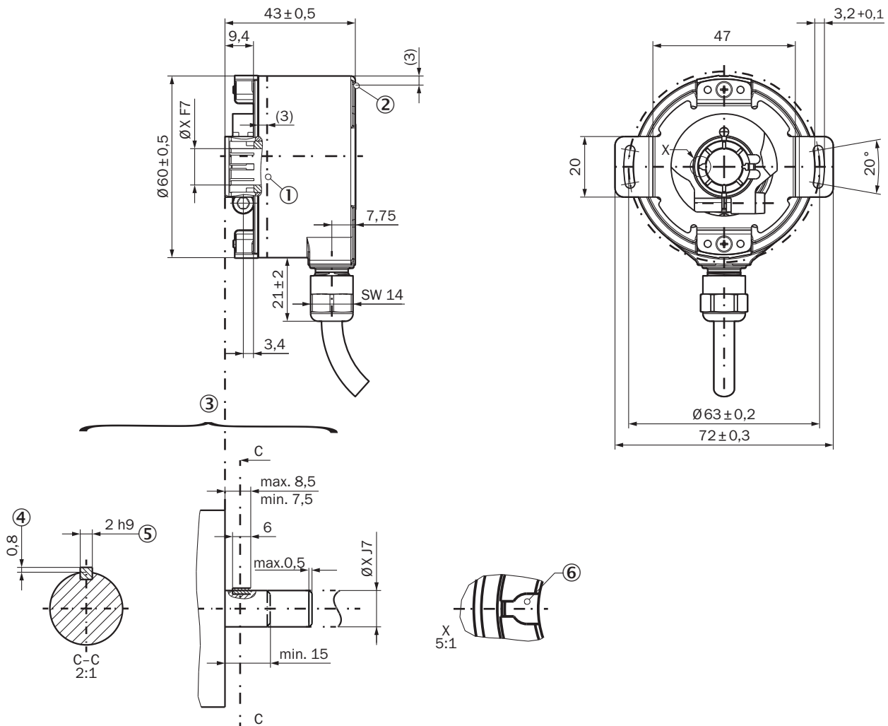
Maßzeichnung Durchsteckhohlwelle, radiale Leitung
